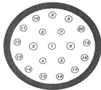
RECEPTACLE ( PIN )
