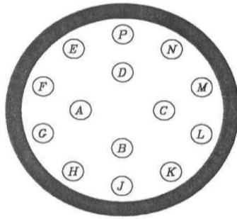
RECEPTACLE ( PIN )
